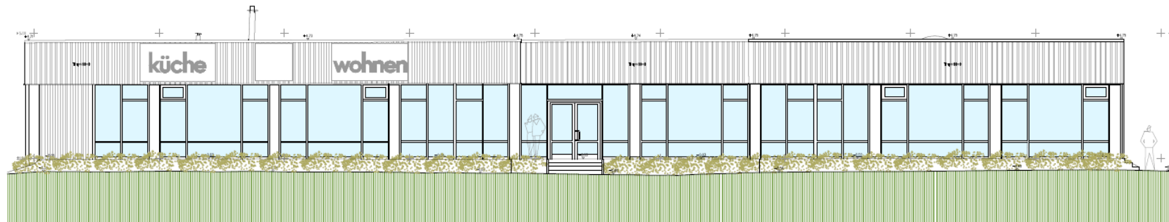
WESTANSICHT:
